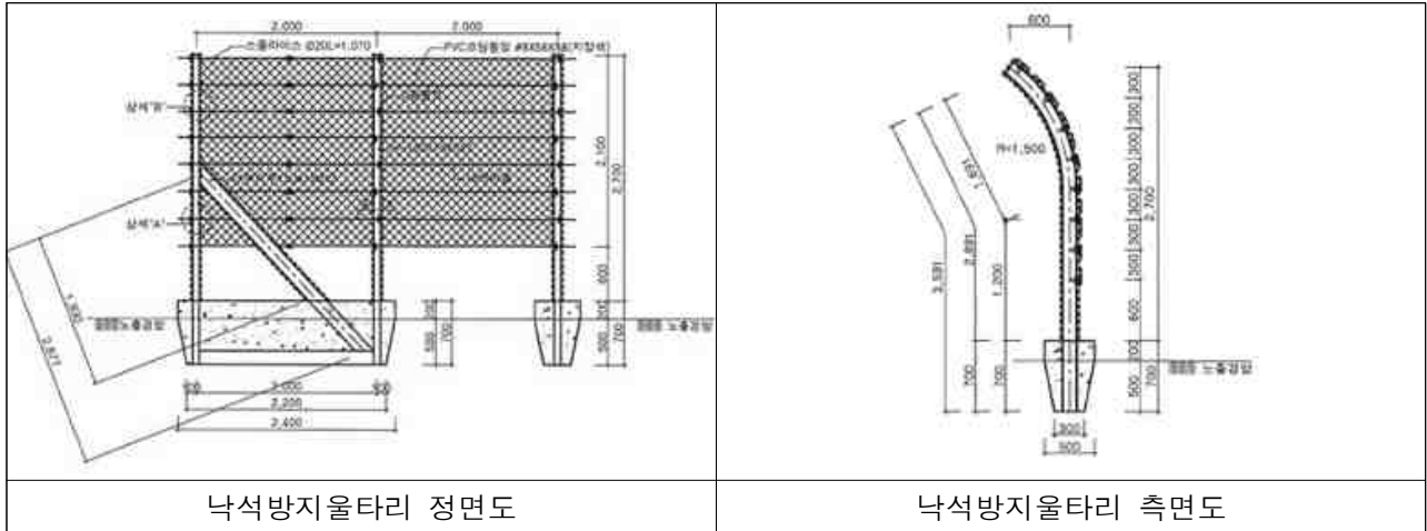
[그림2] 2024년 ○○○○○○○○ 재난취약지구 정비공사 낙석방지울타리 단부구간 현황
